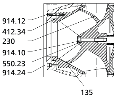
Fig. 10: D impeller
